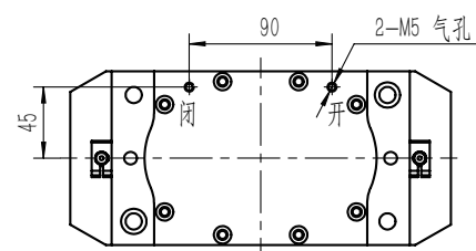
B底部通气款底部气孔尺寸示意
